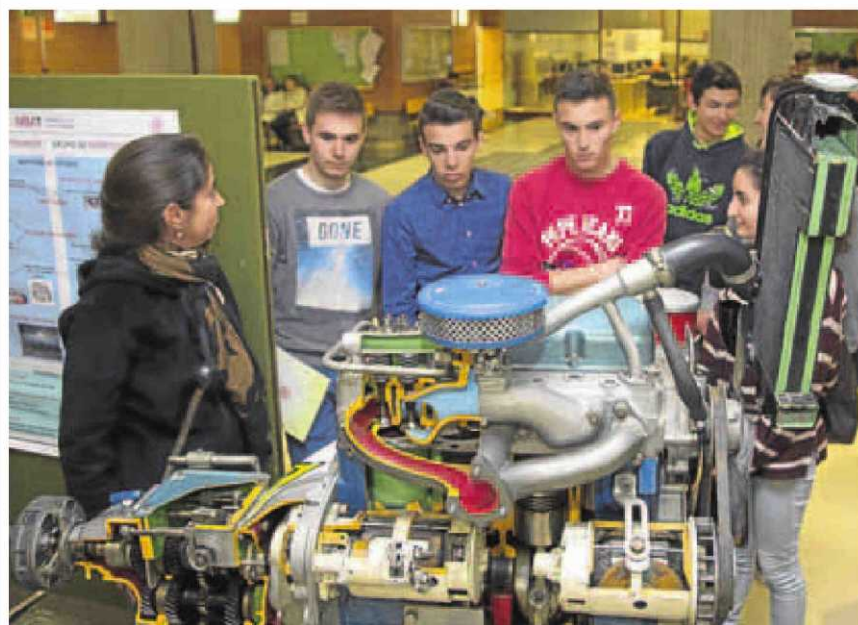
Una profesora muestra el funcionamiento de un motor en la Escuela de Ingenieros.
